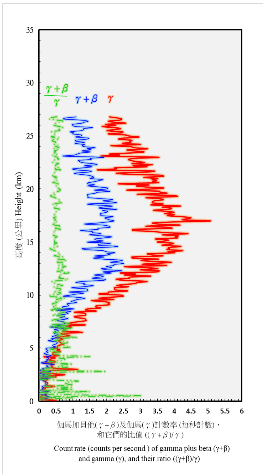
圖 7. 二零二二年內在京士柏進行的高空輻射探測之平均大氣放射性垂直廓線 (探測日期為：六月十三日及九月二十六日)。
