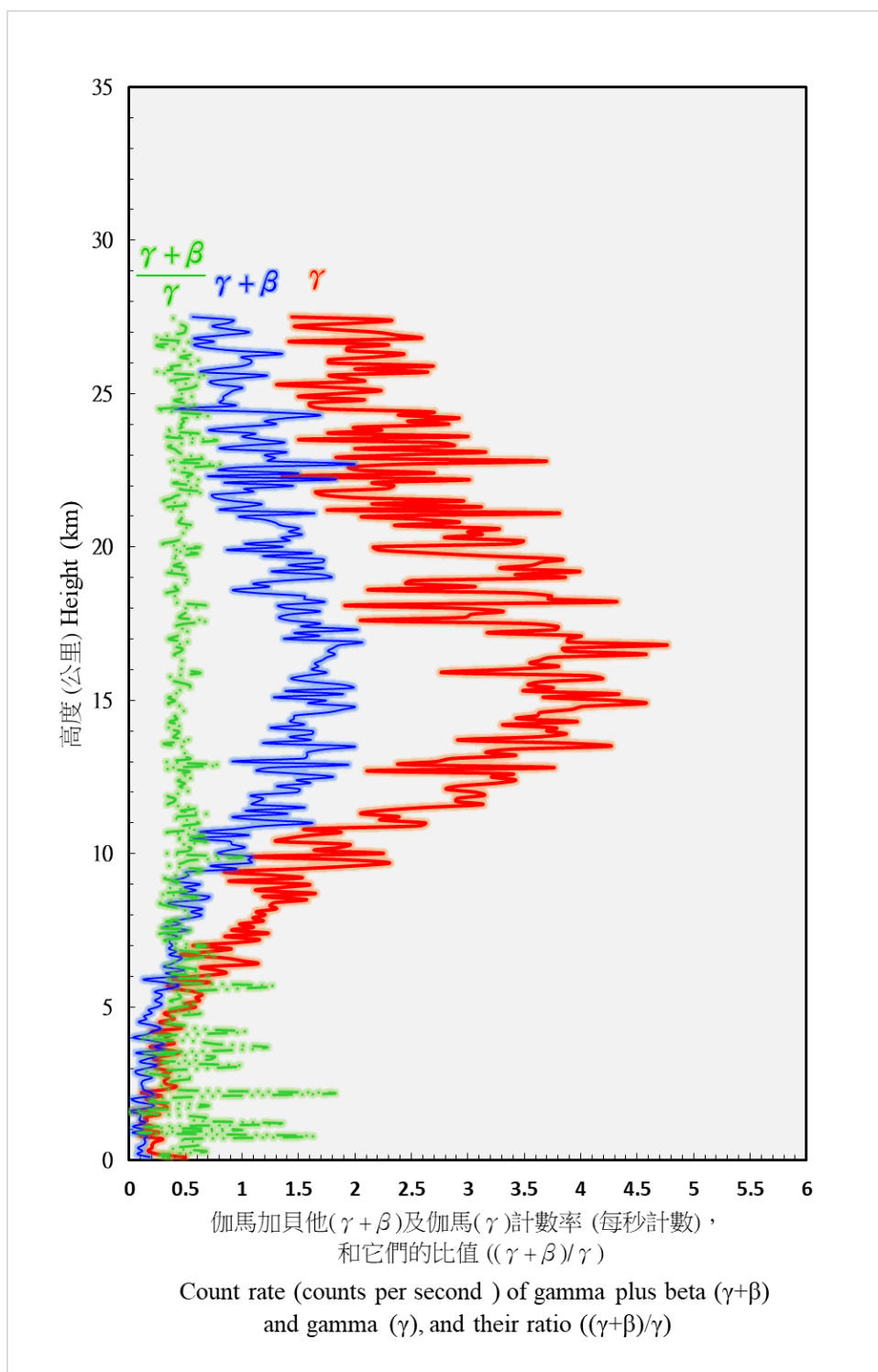
圖 7. 二零二一年內在京士柏進行的高空輻射探測之平均大氣放射性垂直廓線 (探測日期為：五月二十七日及八月二十六日)。
