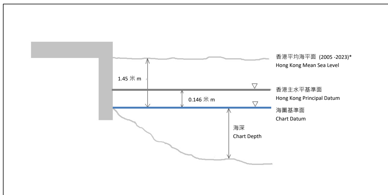
香港高程基準示意圖 Illustration diagram of Hong Kong Vertical Datum
