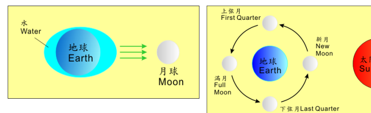
潮汐的示意圖 (不依比例)
